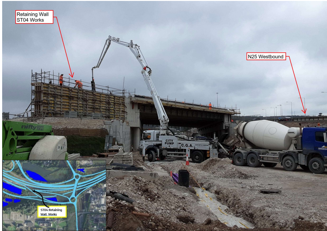
Retaining Wall pour ongoing at Structure ST04
